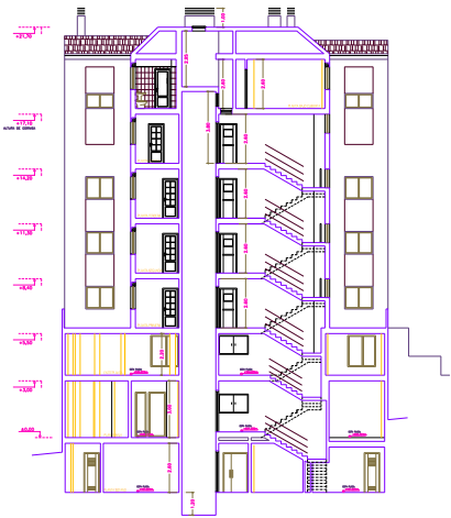
Seccion A-A Escala 1/100
